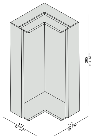
Modulo angolare Corner module
