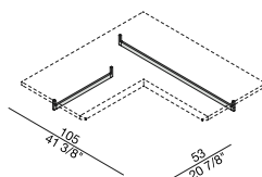
Appendria angolare Corner Hanging bar
