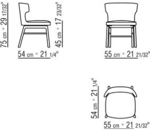
COD. 02B001 CHAIR CANALETTO/OAK FEET
