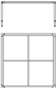
C 87003 Tavolo quadrato in acciaio, 6 doghe Square table in steel, 6 slats cm 162 x 162 x h 73 in 63 7/8 x 63 7/8 x h 28 3/4
