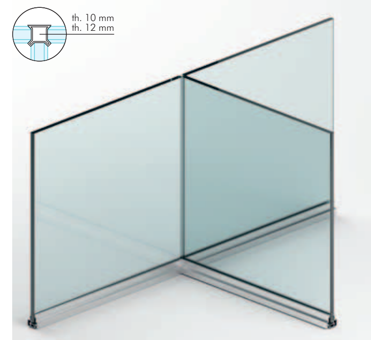
Giunto angolare 3 vie in polycarbonato 90 ° 3-Ways polycarbonate 90° corner joint 3 Wege Eckverbindung aus Polycarbonat 90 ° Jonction angle 3 voies en polycarbonate 90 ° Perfil de conexion en polycarbonato a 3 vias 90 °
