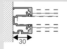
A Elemento di partenza da muro - FISSO Wall starting element - FIXED Maueranschlusselement - FIXED Profil départ pour fixation au mur - FIXÉ Elemento inicial a muro - FIJO
