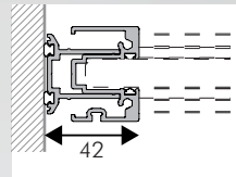
B Elemento di partenza da muro - TELESOPICO Wall starting element - ADJUSTABLE PROFILE Maueranschlusselement - REGULIERBAR PROFIL Profil départ pour fixation au mur - PROFIL RÉGLABLE Elemento inicial a muro - PERFIL AJUSTABLE
