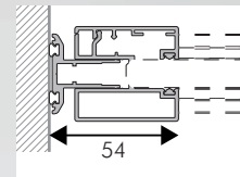
C Elemento di partenza da muro - REGOLABILE Wall starting element - ADJUSTABLE PROFILE Maueranschlusselement - REGULIERBAR PROFIL Profil départ pour fixation au mur - PROFIL RÉGLABLE Elemento inicial a muro - PERFIL AJUSTABLE
