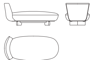
52564 Day bed rivestimento tessuto o pelle (seduta/schienale anche 2 varianti di tessuto) Day bed fabric or leather upholstery (seat/back also in 2 different fabrics) cm 172 x 76 x h 68 in 67 3/4 x 30 x h 26 3/4
