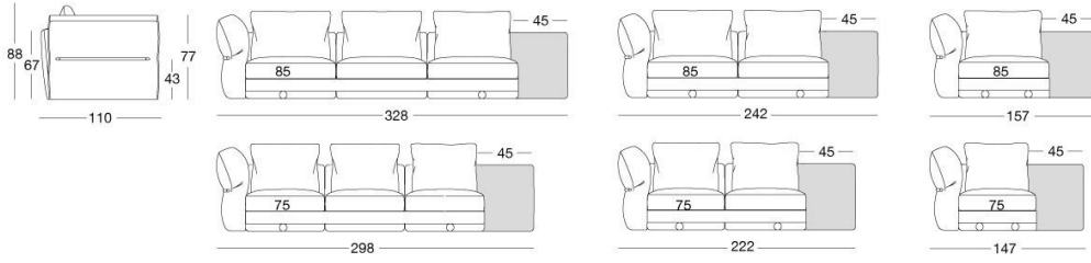
Terminali Dx con schienale allungato / Right end unit with extended back / Боковая секция с удлиненной спинкой правая
