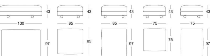
Pouf / Pouf / Пуф
