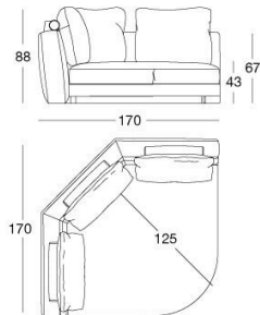
Angolo aperto / Open corner / Открытый угловой элемент
