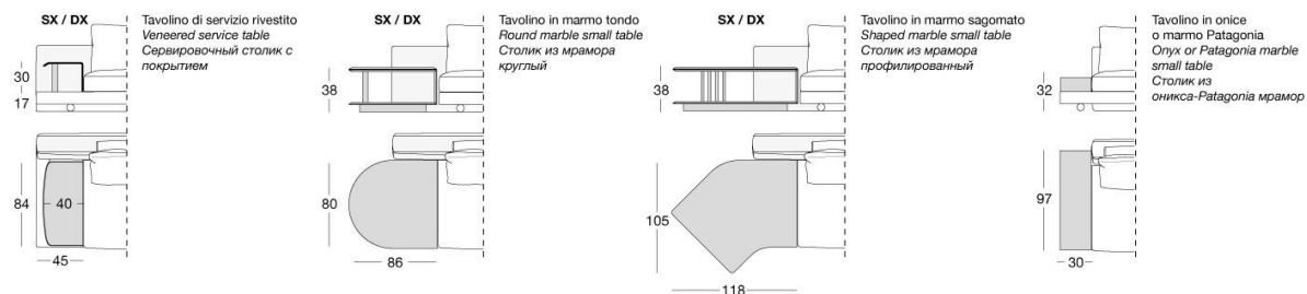
Accessori per elemento terminale / End unit accessories / Аксессуары для боковой секции
